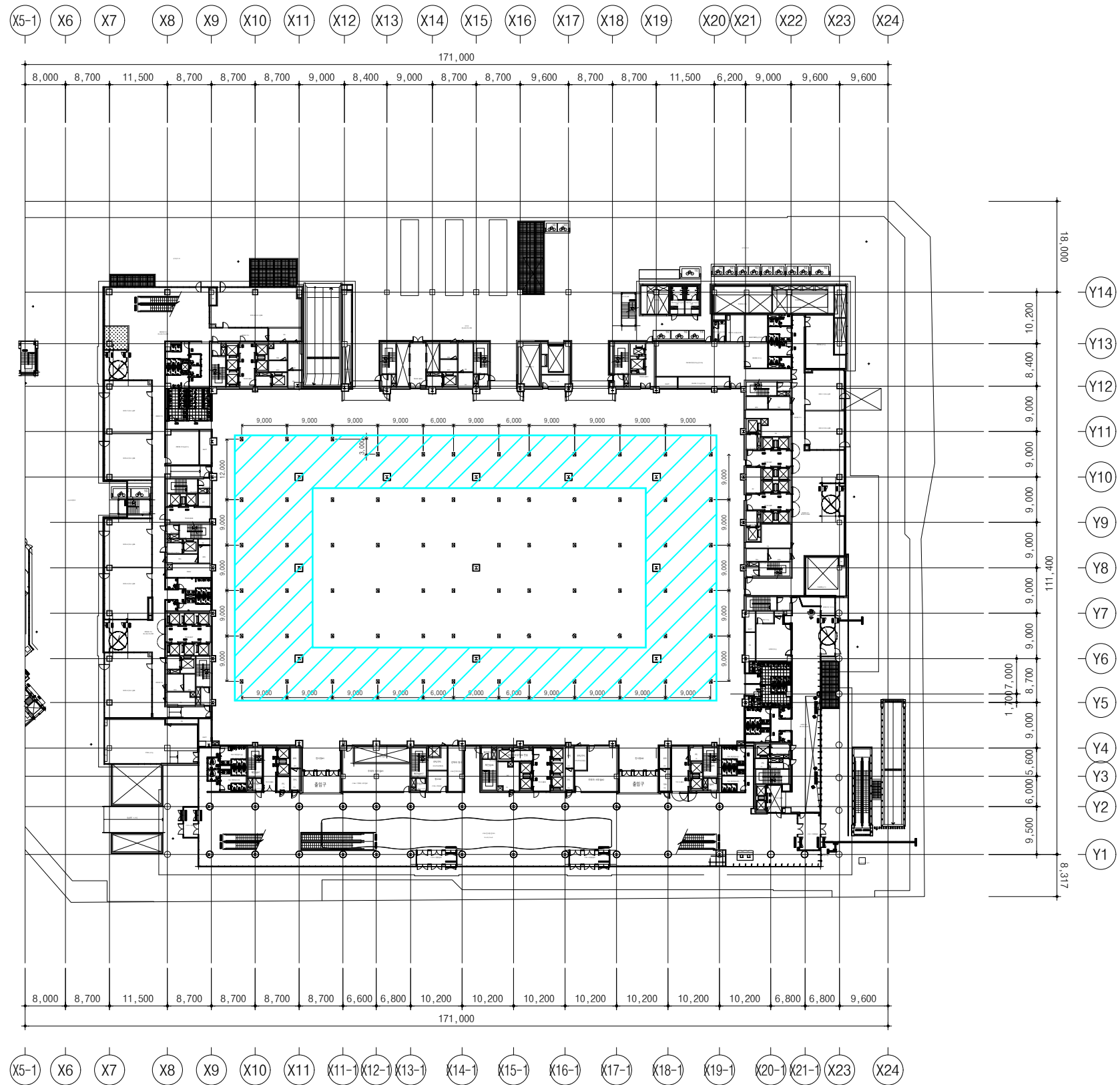
전시홀(급,배수 유틸리티) 평면도
